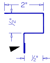
1/2" DOUBLE J ISC-06
