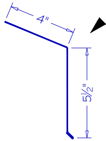
EAVE EV-04
