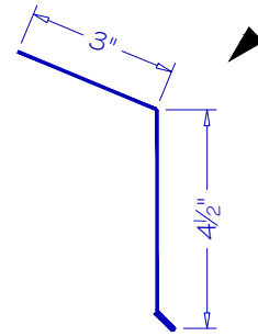
EAVE EV-03
