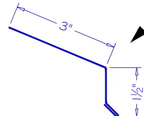
DOOR JAMB DJ-01
