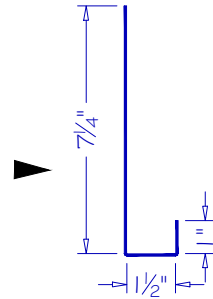
DOOR JAMB DJ-01
