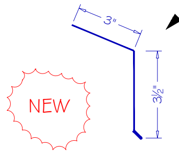
EAVE EV-05
